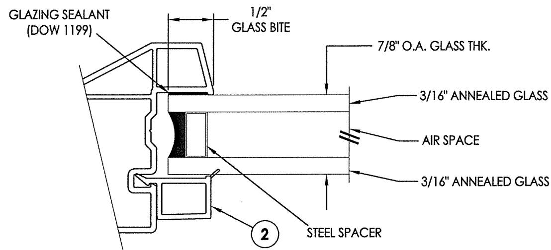
G2 GLAZING DETAIL
